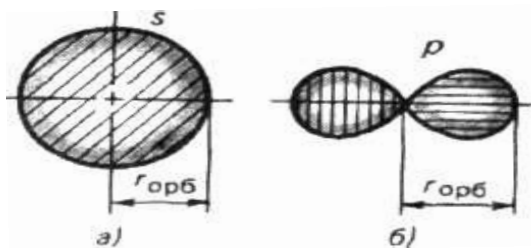
Рисунок 3 – Определение орбитального радиуса r_o для атомных орбиталей разной формы: a – s -орбиталь; b – p -орбиталь
