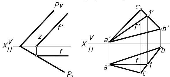
Рисунок 4.8 – Фронталь плоскости
