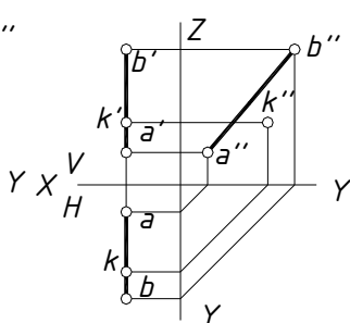
Рисунок 4.3 – Точка не лежит на прямой
