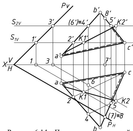
Рисунок 6.14 – Пересечение плоскостей, заданных различными способами
