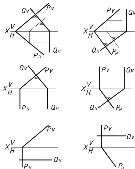
Рисунок 7.12 – Взаимно перпендикулярные плоскости
