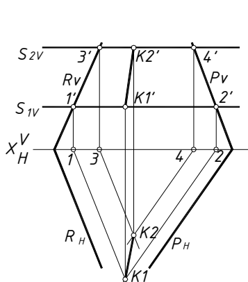
Рисунок 6.13 – Пересечение плоскостей, заданных следами
