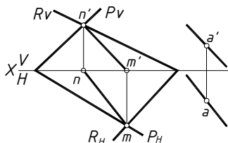
Рисунок 7.2 – Прямая, параллельная двум плоскостям
