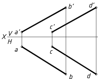
Рисунок 5.1 – Параллельные прямые
