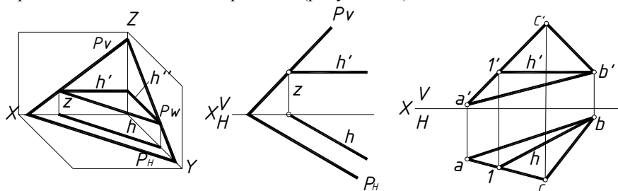
Рисунок 4.7 – Горизонталь плоскости
