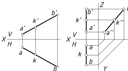
Рисунок 4.2 – Точка принадлежит прямой
