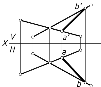
Рисунок 4.4 – Прямая принадлежит плоскости
