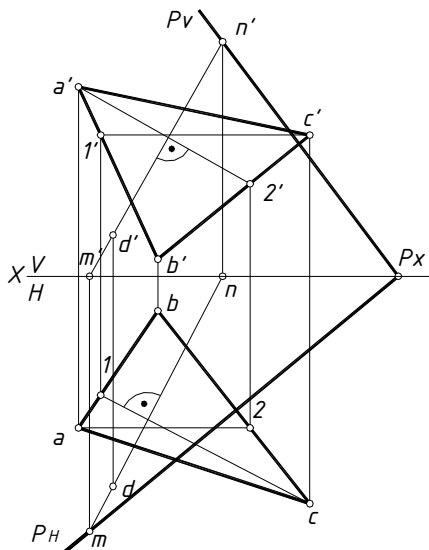
Рисунок 7.10 – Взаимно перпендикулярные плоскости
