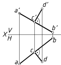
Рисунок 7.7 – Прямые не перпендикулярны между собой
