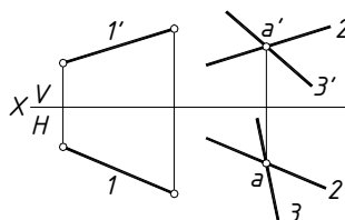
Рисунок 7.3 – Плоскость, параллельная прямой
