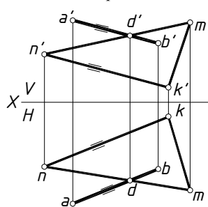
Рисунок 4.5 – Прямая принадлежит плоскости
