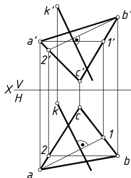
Рисунок 7.8 – Перпендикуляр к плоскости, заданной треугольником
