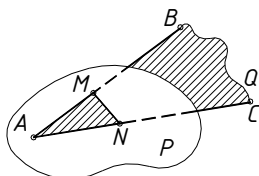
Рисунок 6.3 – Общий принцип построения линии пересечения двух плоскостей
