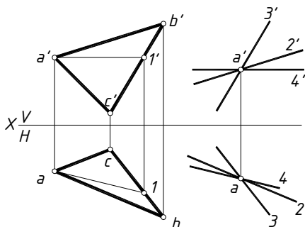
Рисунок 7.1 – Прямая, параллельная плоскости
