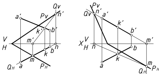
Рисунок 6.8 – Пересечение прямой с плоскостью общего положения, заданной следами
