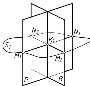
Рисунок 6.12 – Метод плоскостей-посредников
