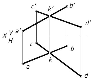
Рисунок 5.3 – Пересекающиеся прямые
