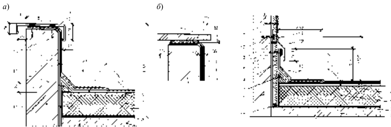
Рисунок 32 – Примыкание двухслойной кровли с выводом на парапет:
