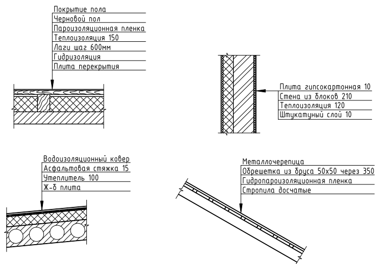
Рисунок 74 – Выносные надписи к многослойным конструкциям
