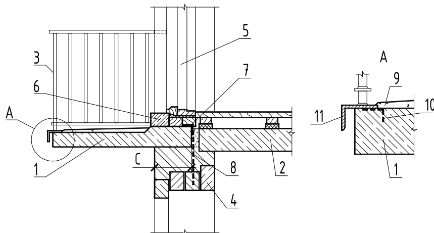
Рисунок 55 – Устройство балкона:
