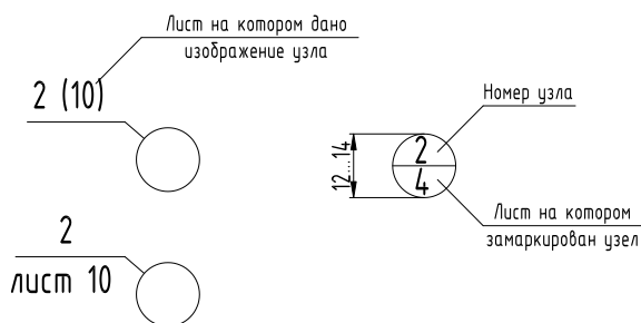
Рисунок 72 – Маркировка выносного элемента
