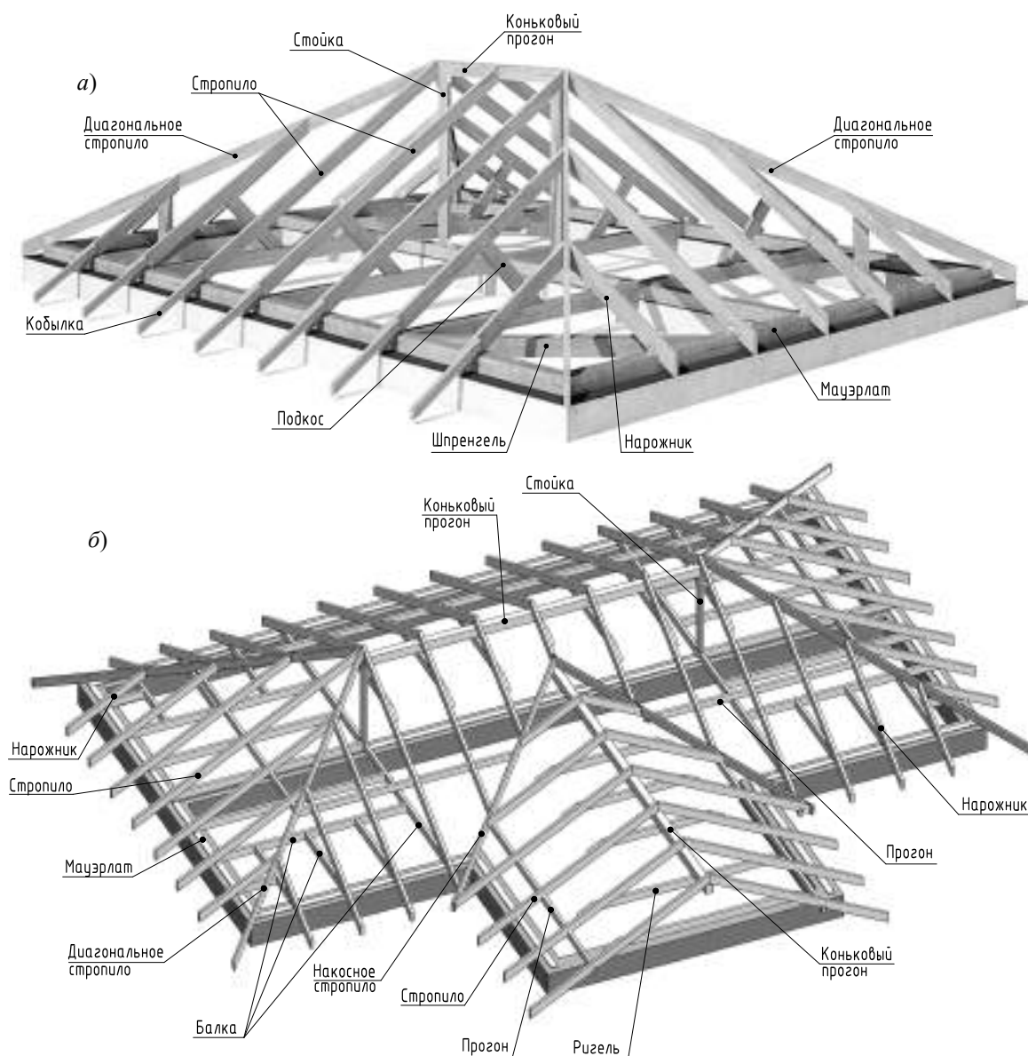
Рисунок 20 – Примеры стропильных систем: а – вальмовая крыша; б – многоскатная крыша
