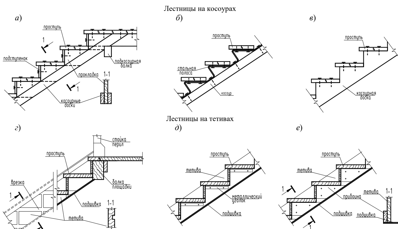
Рисунок 41 – Варианты конструктивного исполнения деревянной лестницы:
