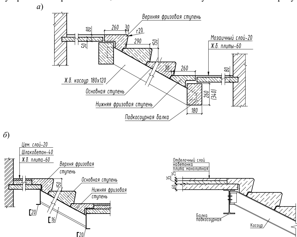
Рисунок 51 – Варианты устройства лестницы из железобетонных ступеней: а – на железобетонной подкосоурной балке; б – на металлической подкосоурной балке
