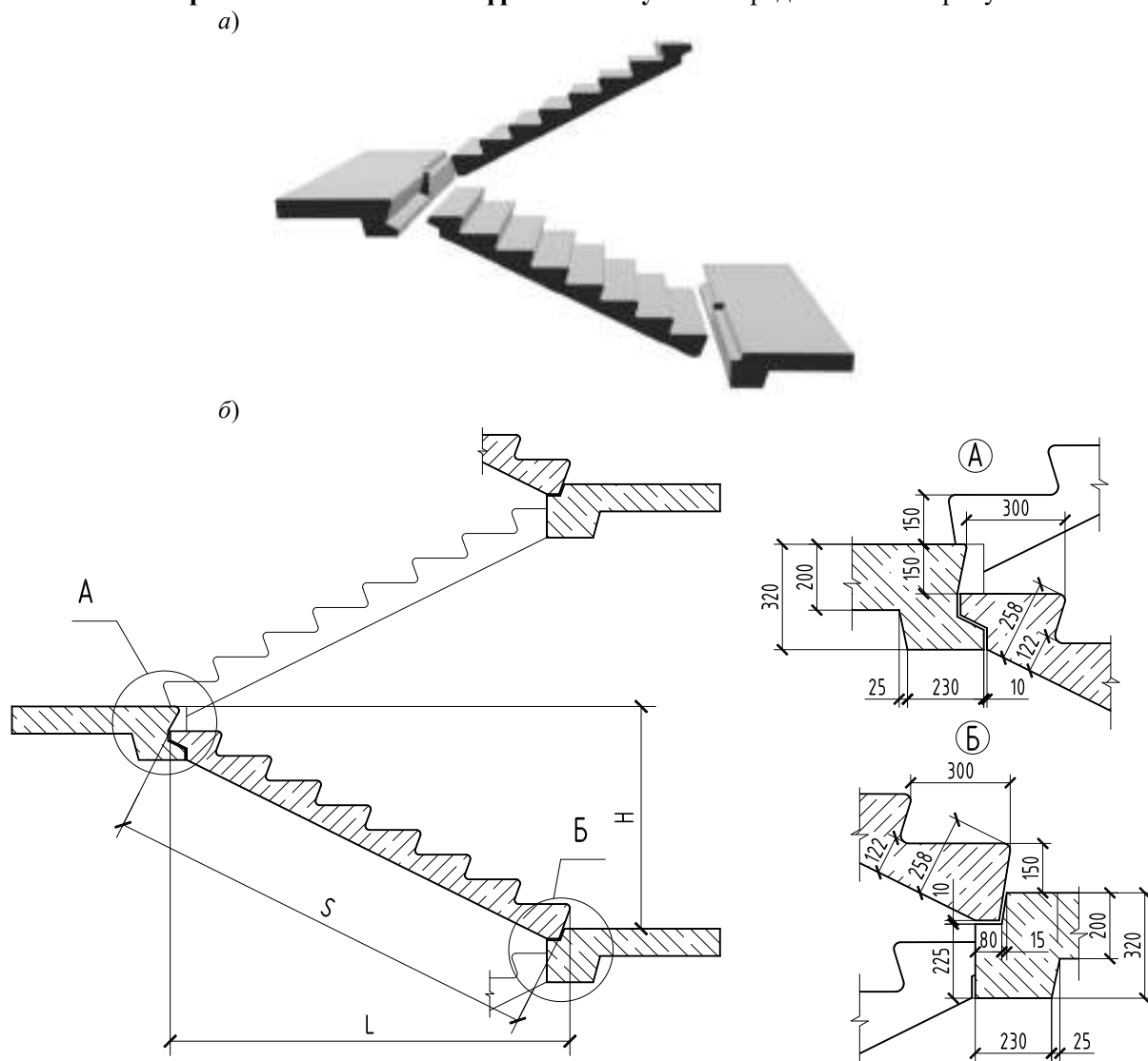
Рисунок 42 – Сборные (плоские) железобетонные лестницы, применяемые в зданиях с поперечными несущими стенами. Лестничный марш ЛМ (плоский без фризových ступеней), площадка 1ЛП:
