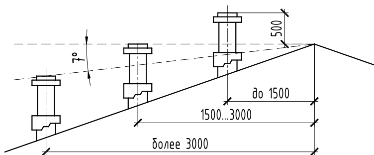
Рисунок 29 – Высота дымовых труб в зависимости от расстояния от конька
