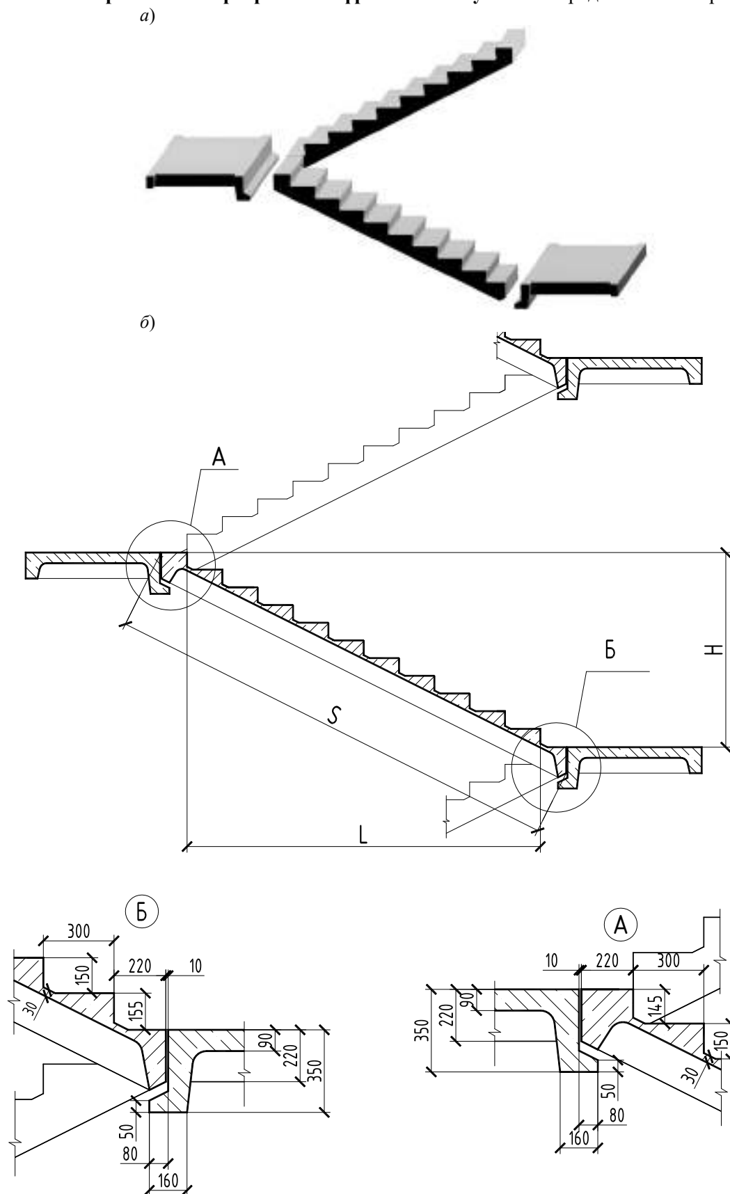
Рисунок 45 – Сборные ребристые железобетонные лестницы, применяемые в зданиях с поперечными несущими стенами. Лестничный марш ЛМФ (с фризowymi ступенями), площадка ЛПФ: а – общий вид; б – изображение в разрезе
