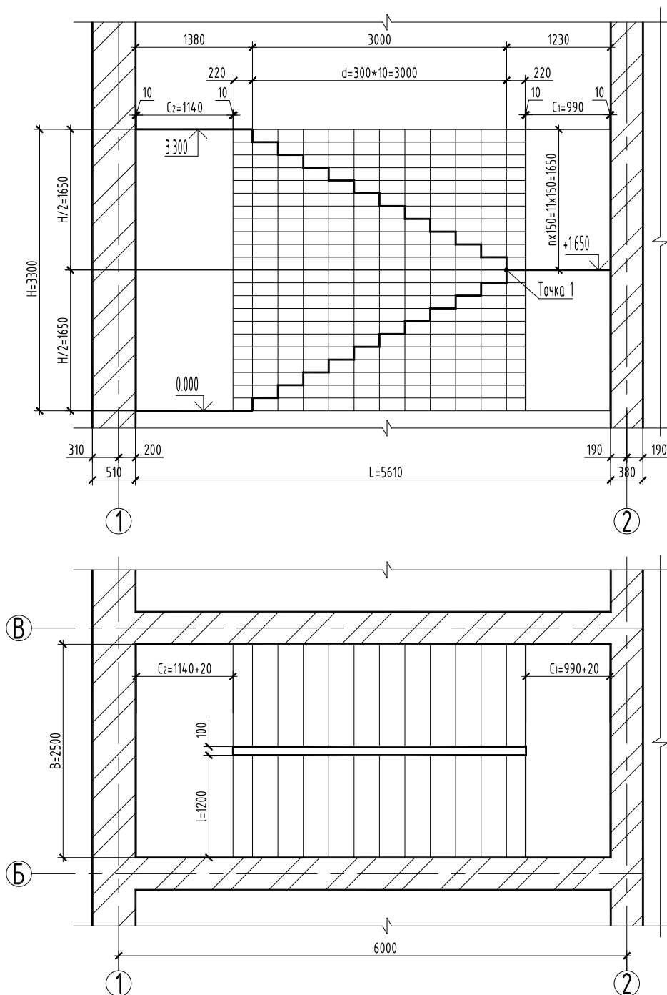
Рисунок 54 – Пример графического расчета лестничного марша
