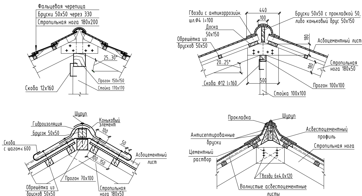
Рисунок 23 – Варианты устройства конькового узла
