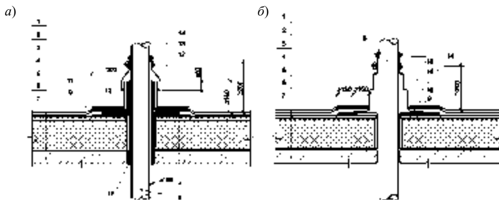
Рисунок 36 – Варианты пропуска труб через кровлю:
