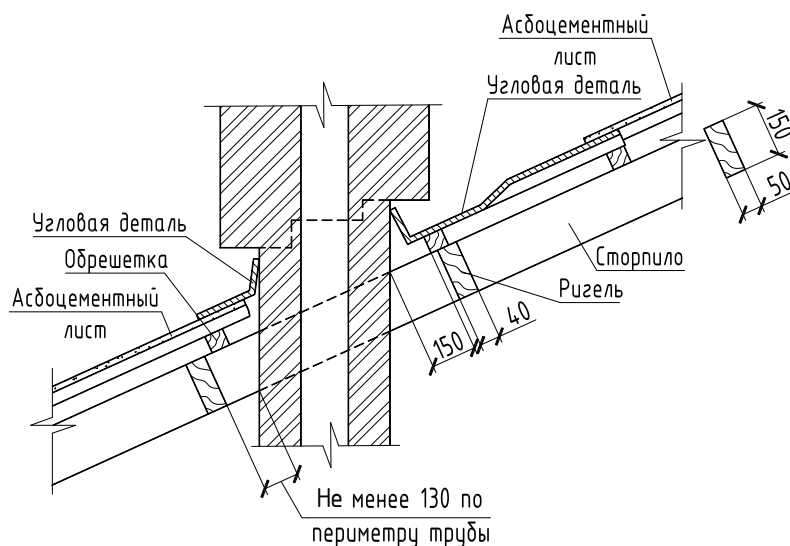
Рисунок 30 – Вариант устройства прохода в кровле под дымовую трубу
