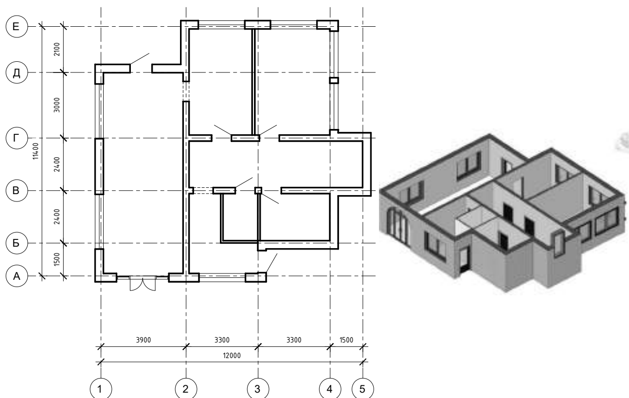
Рисунок 83 – Размещение окон, дверей и перегородок
