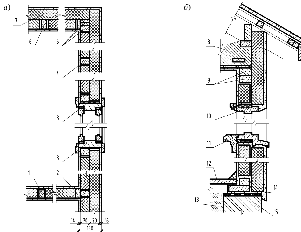
Рисунок 12 – Конструкция стен каркасного дома:
