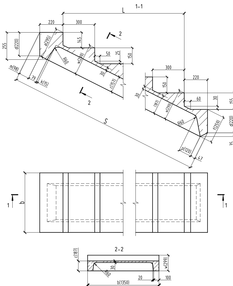
Рисунок 46 – Лестничный марш ЛМФ с фризowymi ступенями (в скобках даны размеры для маршей ЛМФ39 и ЛМФ42)
