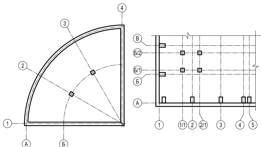
Рисунок 68 – Нанесение координационных осей
