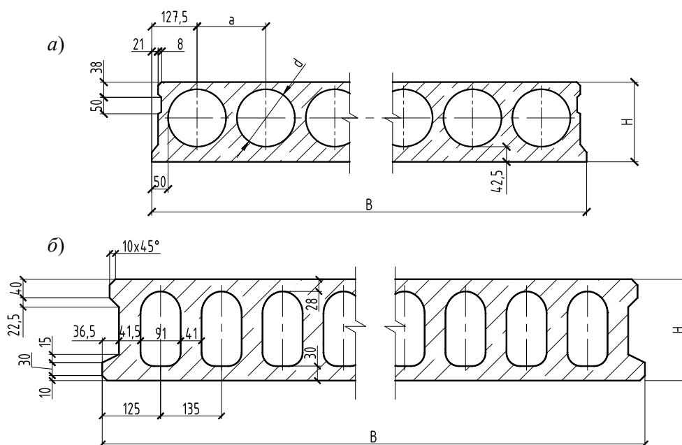
Рисунок 5 – Форма многопустотных плит (СТБ 1383-2003, ГОСТ 9561-16):
