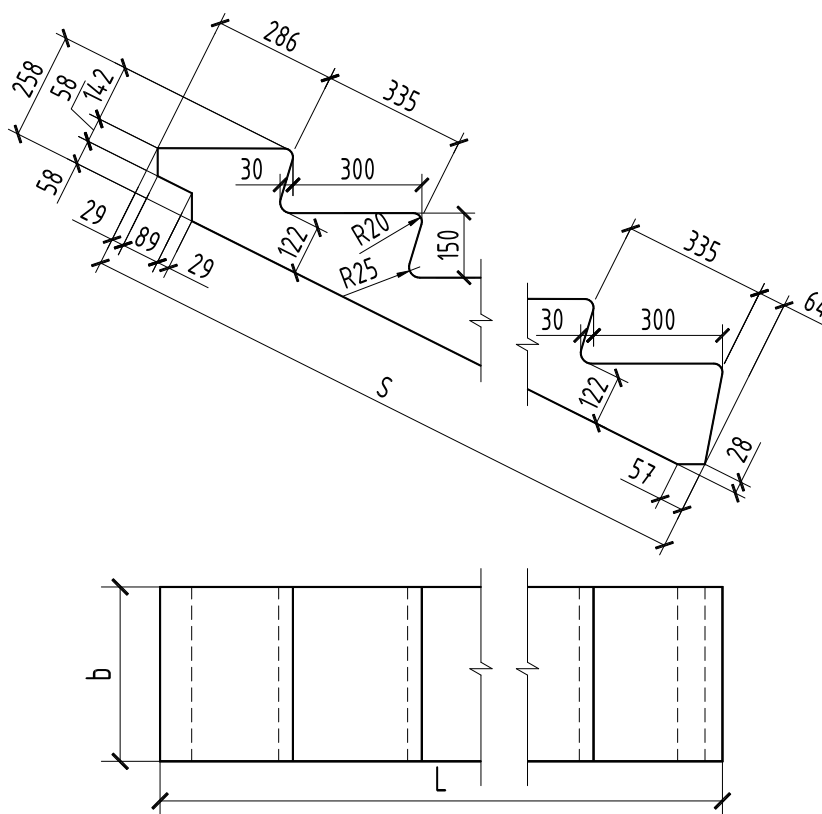
Рисунок 43 – Лестничный марш ЛМ (плоский без фризových ступеней)
