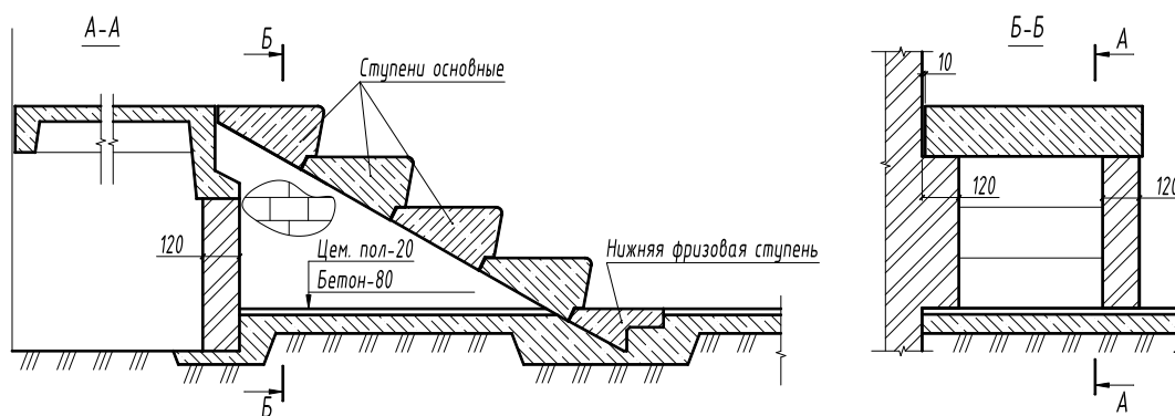
Рисунок 52 – Вариант устройства пригласительного цокольного марша
