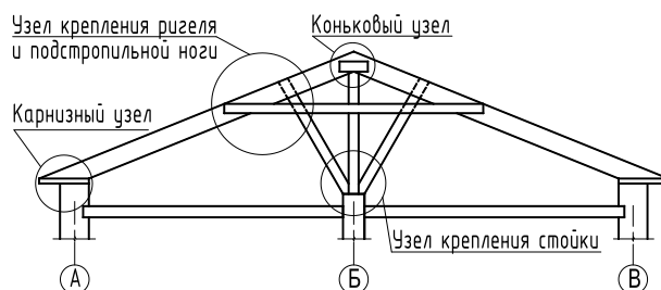
Рисунок 22 – Схема разреза крыши
