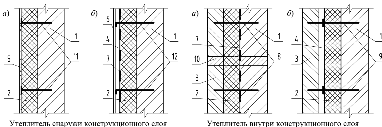
Рисунок 10 – Основные конструктивные решения утепленных наружных стен:
