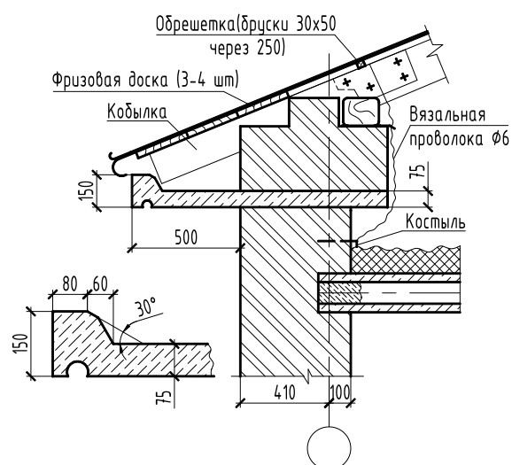
Рисунок 27 – Варианты устройства карнизного узла
