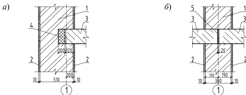
Рисунок 9 – Однослойная каменная стена без утепления:
