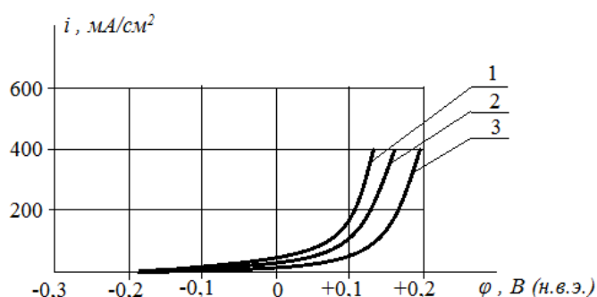
Рисунок 1 – Анодные потенциодинамические поляризационные кривые
