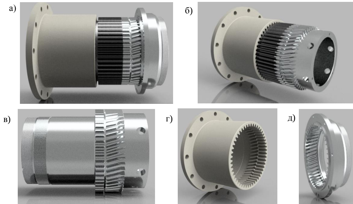
Рисунок 2 – 3D модель тангенциально-осевого замка: а), б) тангенциально-осевой замок; в) втулка неподвижная; г) втулка подвижная; д) муфта замковая
